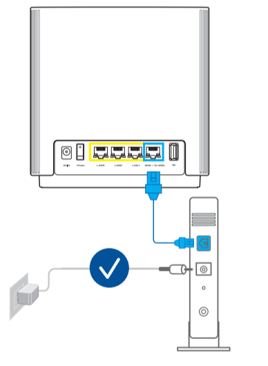
Parte posterior del módem
