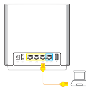
Parte posterior del módem
